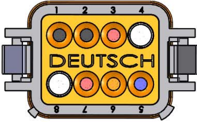
0857-1 Current Sense
